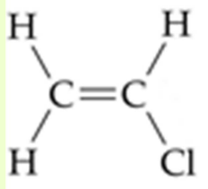
Obrázek 1: Vinylchlorid
