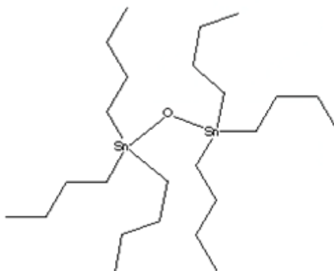
Obrázek 1: Struktura oxidu tri- n -butylcínového
