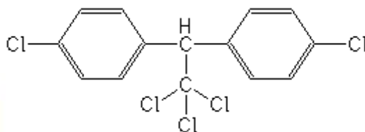
Obr. 1. Molekula DDT
