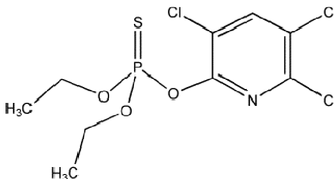
Obrázek 1: Struktura chlorpyrifosu
