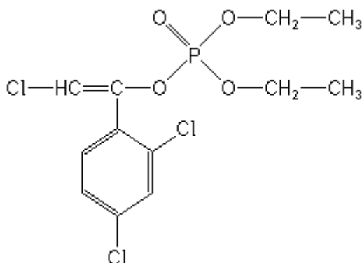
Obrázek 1: Struktura chlorfenvinfosu
