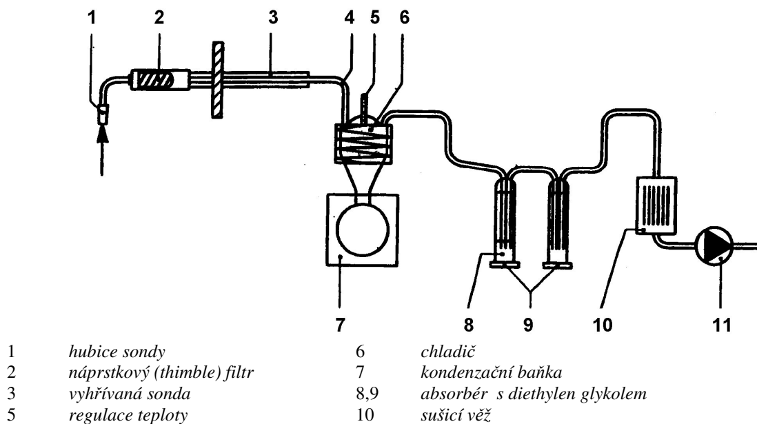
Obrázek 1 Vzorkovací trať pro stanovení PAH – metoda filtračně-kondenzační s vyhřívávanou sondou (ISO 11338-1)
