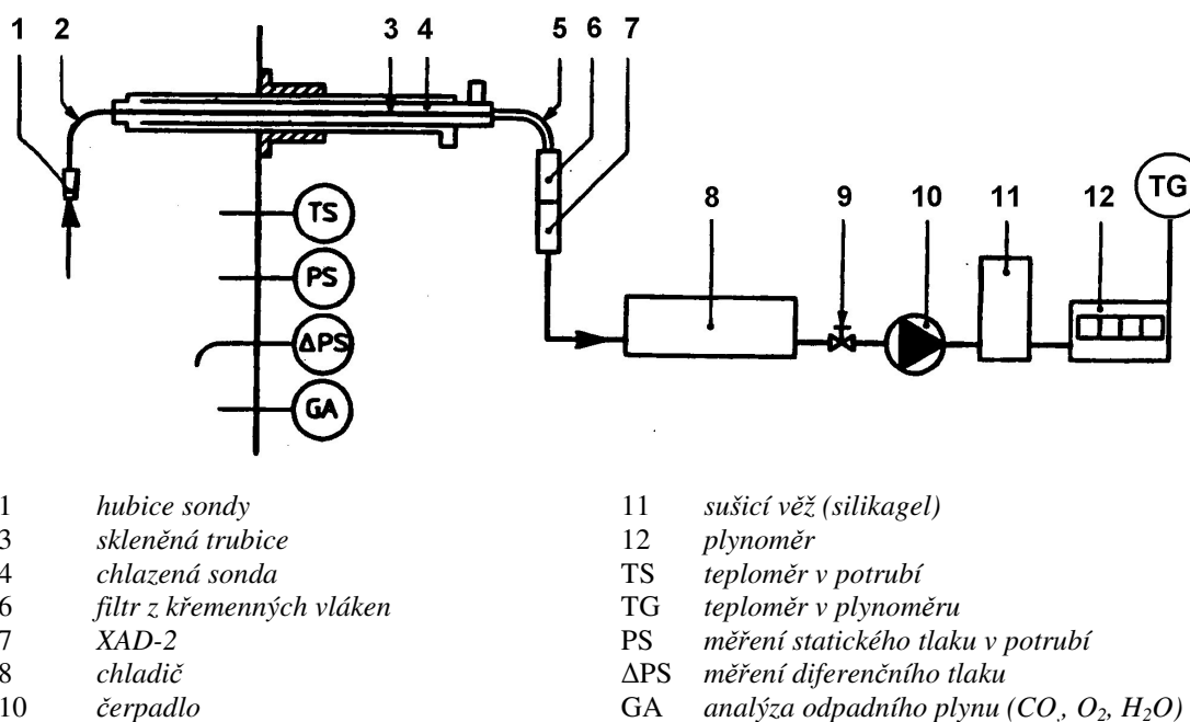
Obrázek 2 Vzorkovací trať pro stanovení PAH - metoda filtračně-kondenzační s chlazenou sondou (ISO 11338-1)
